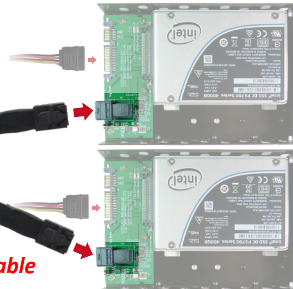
Model No.: PA417G 3.5" Mini SAS HD & SATA to U.2 / SAS / SATA SSD Adapter
